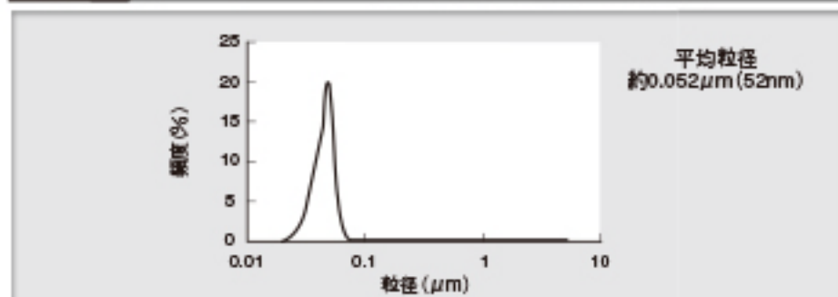
グラフ2 「コエンザイムQ 10 10%水溶化液」の粒度分布(水分散時)
