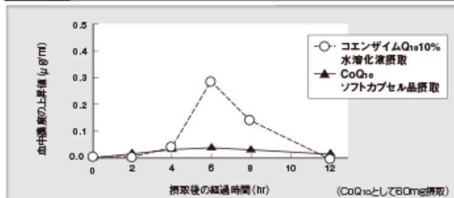
グラフ1 空腹時における「コエンザイムQ 10 10%水溶化液」摂取後の血中濃度上昇推移(成人男子)
